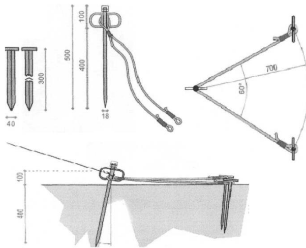
Способ крепления конца леера.
